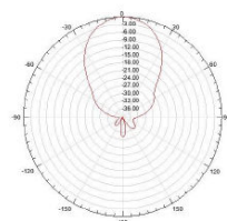
3300-3800MHz
